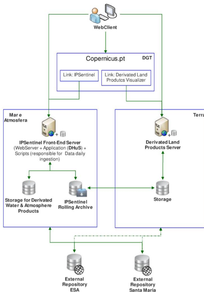
Figura 2 – Arquitetura IPSentinel
